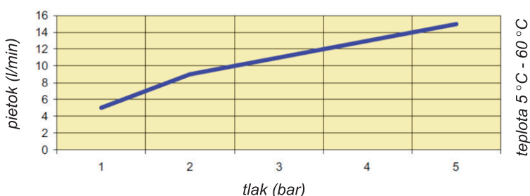
graf závislosti prietoku a tlaku
