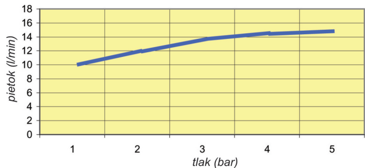
graf závislosti prietoku a tlaku
